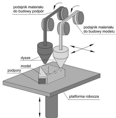
Technologia RP tzw. wytłaczania warstw stopionego polimeru
