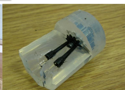
Komora próżniowa i widok elementów przekładni robota kuchennego odlanych w formie silikonowej
