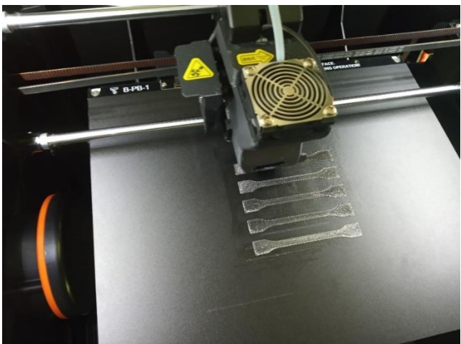
Technologia RP tzw. wytłaczania warstw stopionego polimeru
