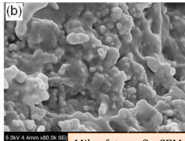
Mikrofotografie SEM kruchych przełomów: EP z 3,0% dodatkiem I-HS-P3 (a) oraz EP z 4,5% dodatkiem I-HS-P3 (b).
