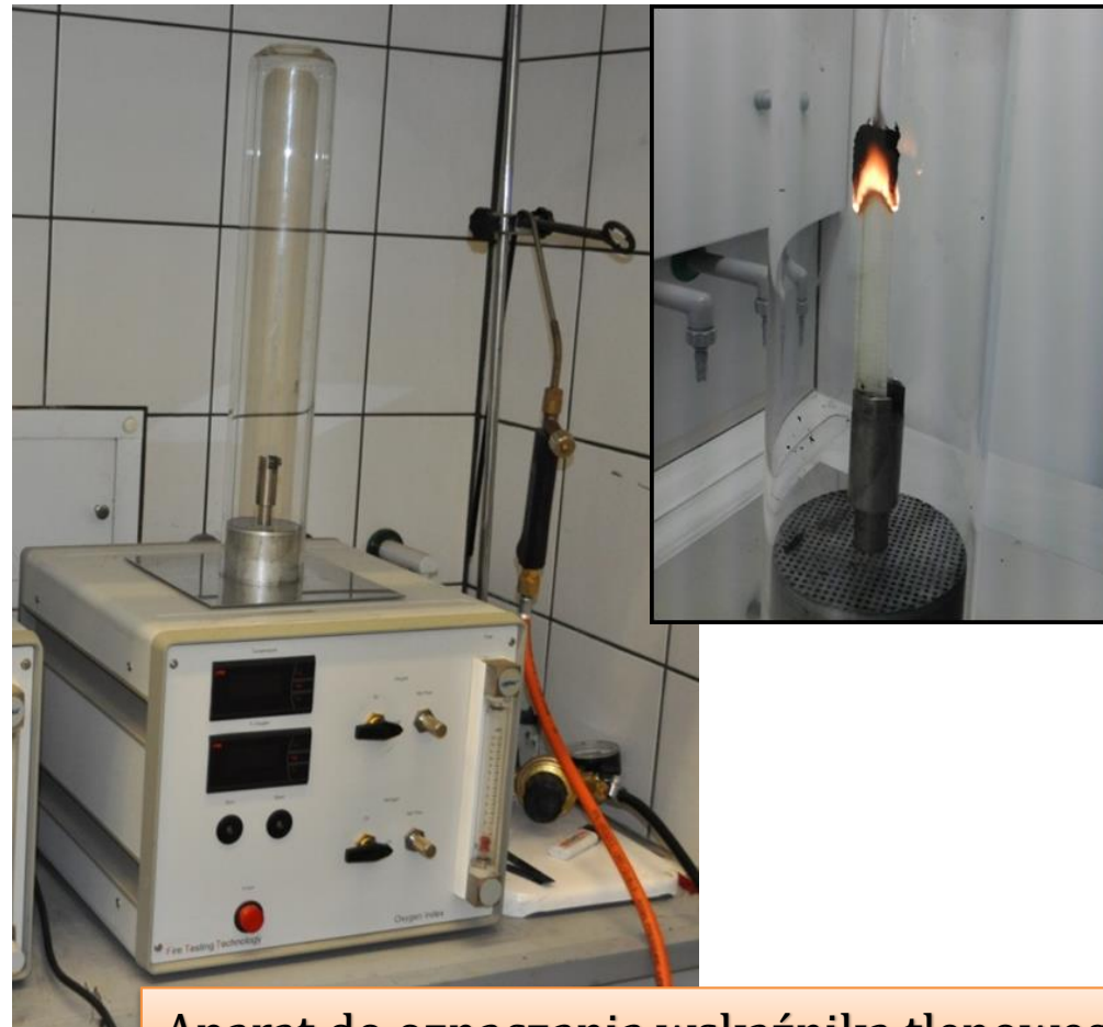
Aparat do oznaczania wskaźnika tlenowego LOI FFT
